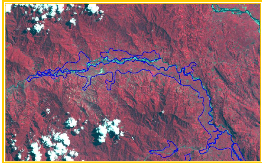
Figura 23. Fondo de valle fluvial
