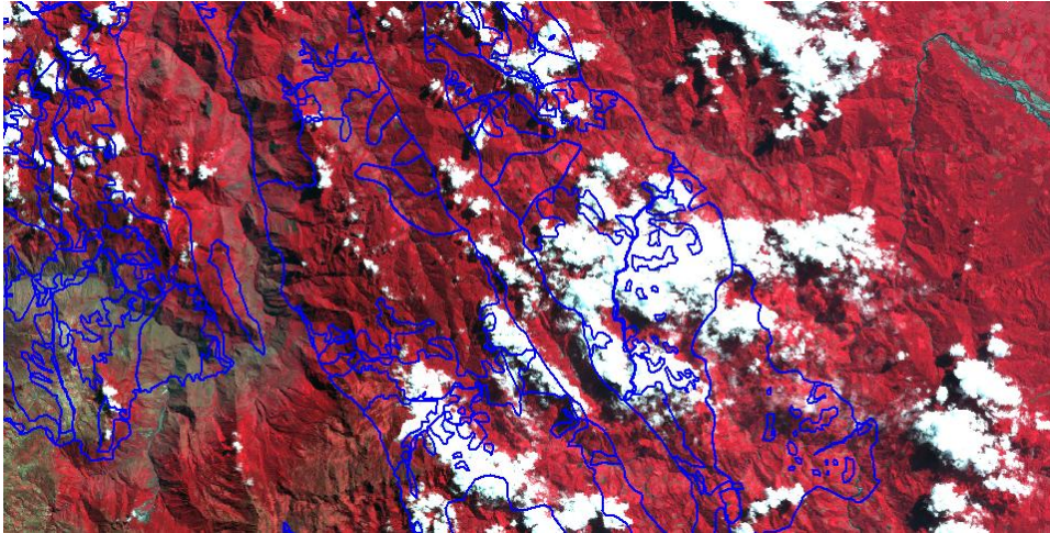
Figura 6. Montañas calcáreas
