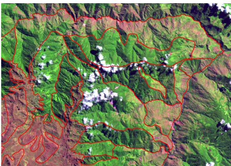
Figura 7. Montañas estructurales plegadas
