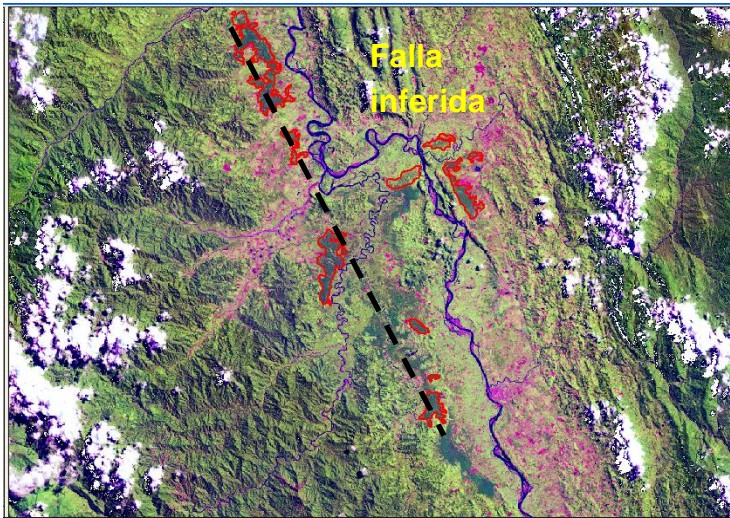
Figura 14. Cubeta fluvio-lacustre y palustre
