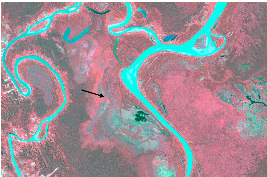
Figura 14. Cubeta fluvio-lacustre y palustre ( Amazónica)
