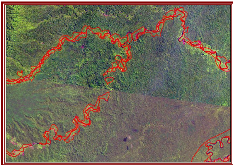
Figura 12. Llanura de inundación fluvial
