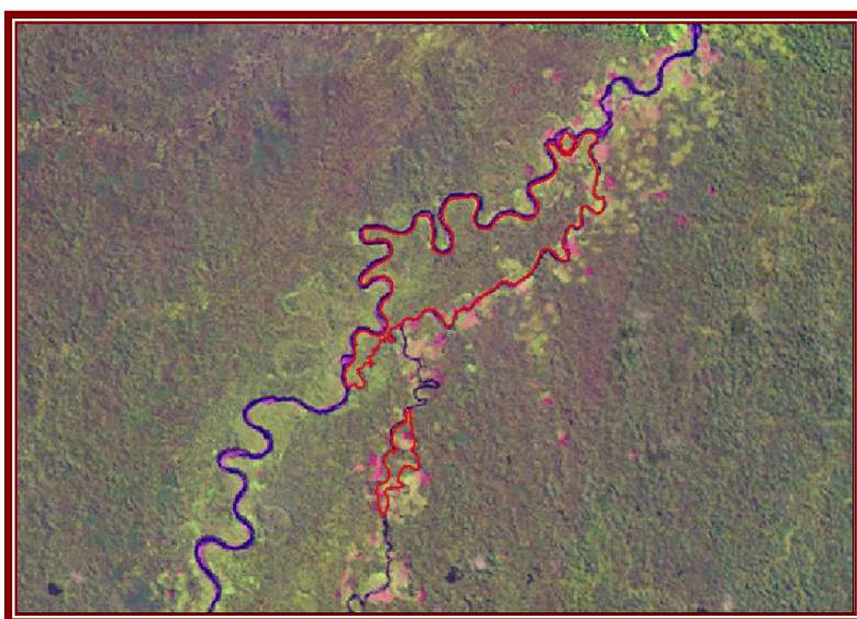
Figura 11. Islas
