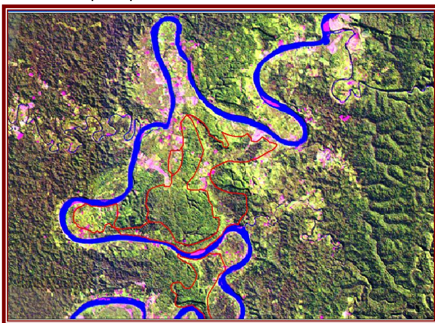
Figura 17. Planicie erosiva antigua (pleistocénica)
