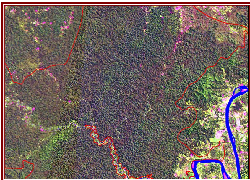
Figura 19. Colinas erosionales del Cuaternario
