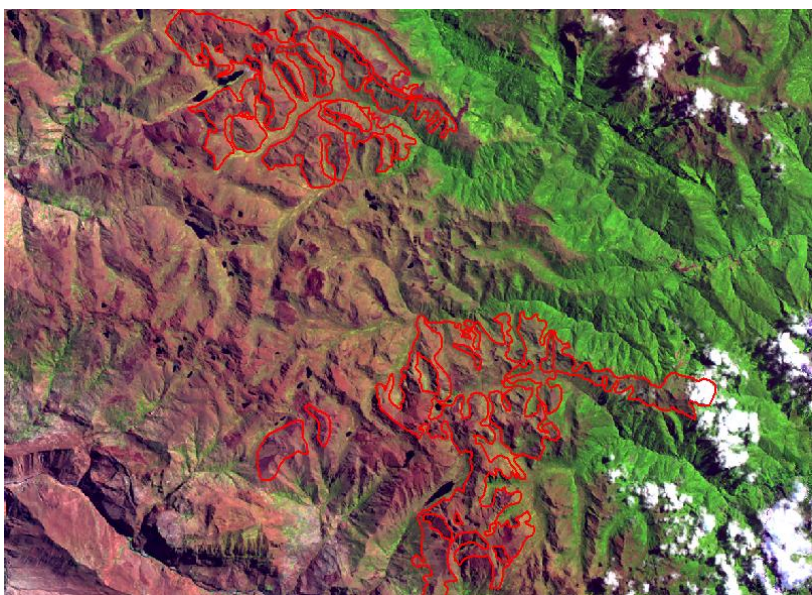
Figura 3. Montañas metamórficas
