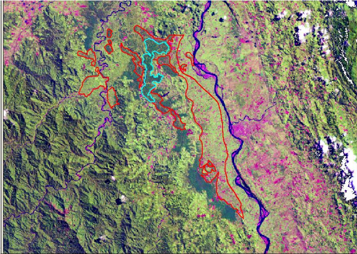
Figura 13. Llanura no inundable subreciente.
