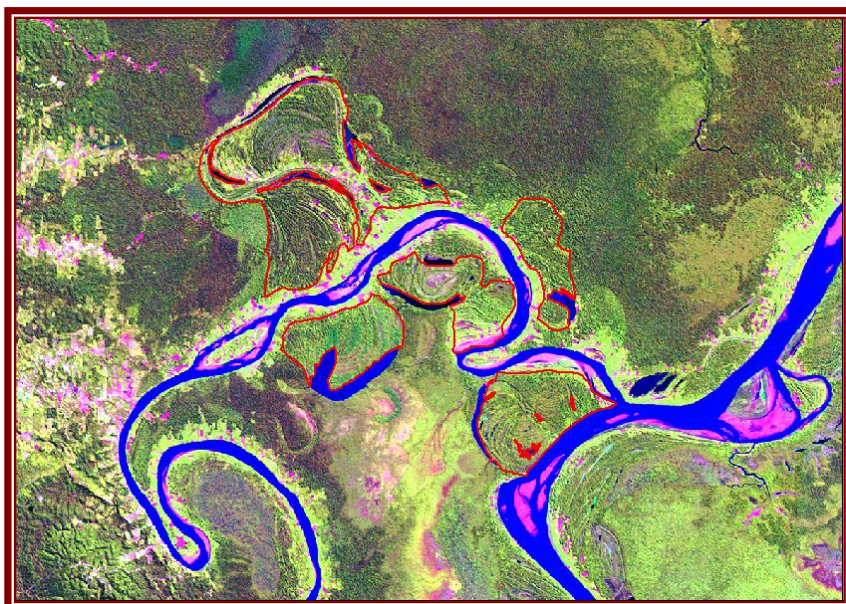
Figura 9. Barras laterales y semilunares
