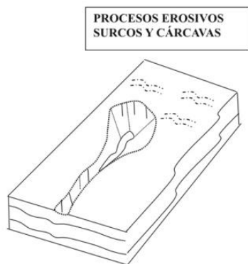
Figura 21. Procesos erosivos en cárcavas
