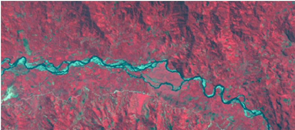
Figura 11. Islas ( Islas Subandinas)
