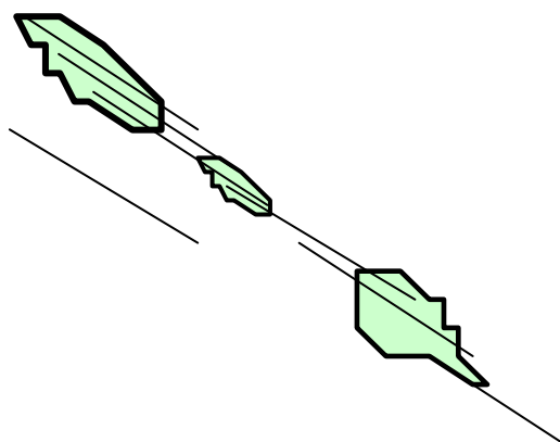
Figura 15. Cubetas lacustres de origen endógeno
