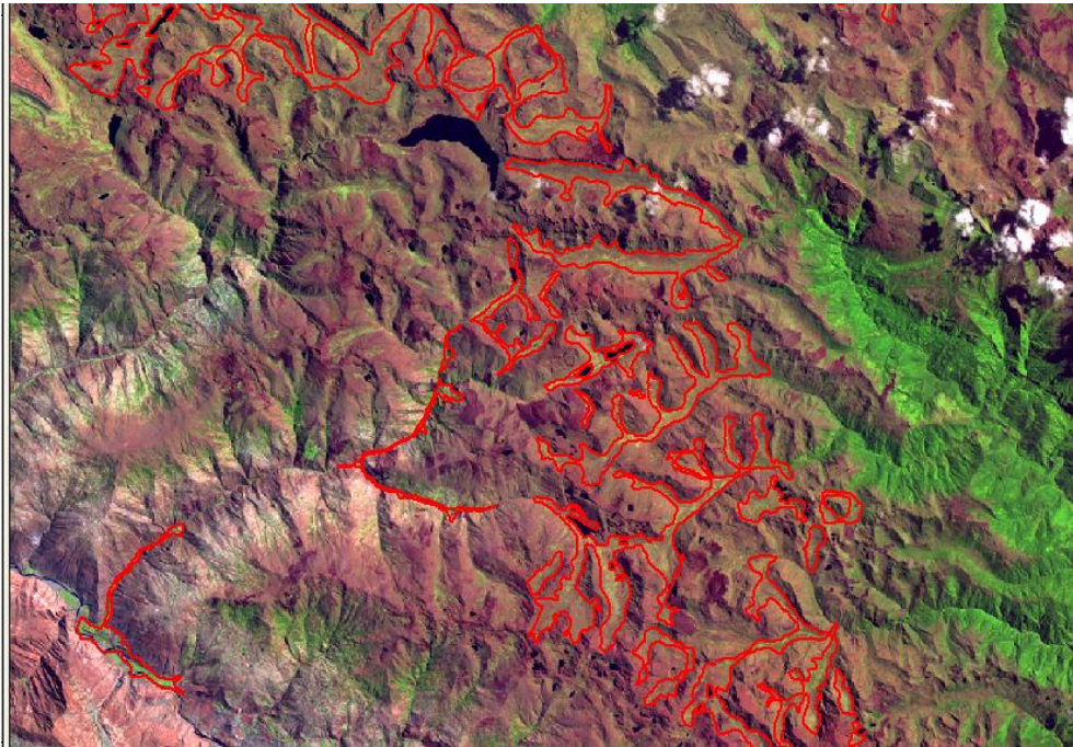
Figura 5. Valles glaciares
