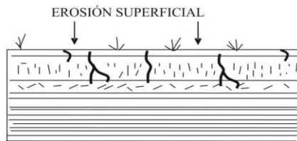
Figura 18. Erosión superficial
