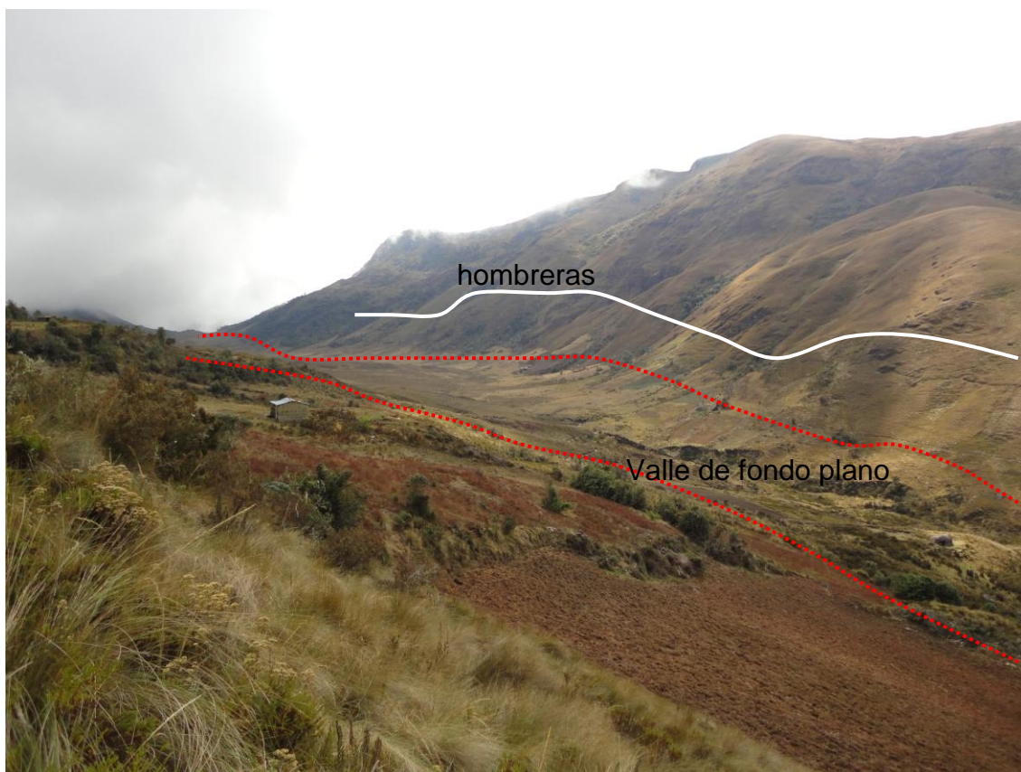
Foto 1. Valle glaciario Bombón. Cercanías de Huanuco. Julio de 2010
