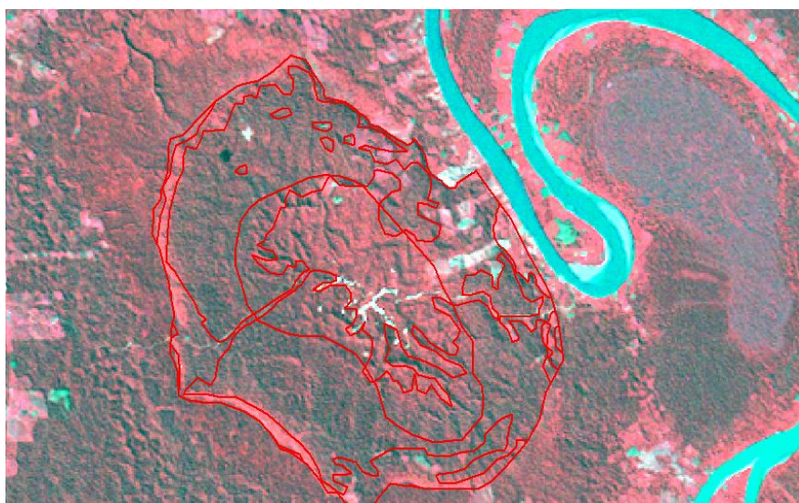
Figura 8. Domo
