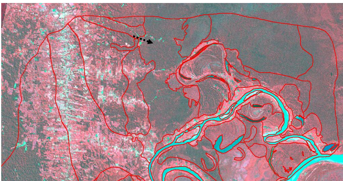
Figura 13. Llanura no inundable subreciente.
