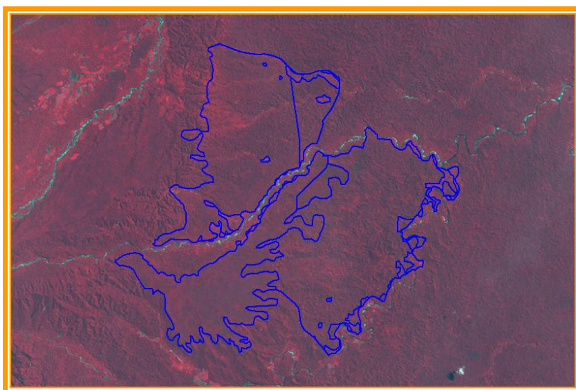
Figura 22. Glacís
