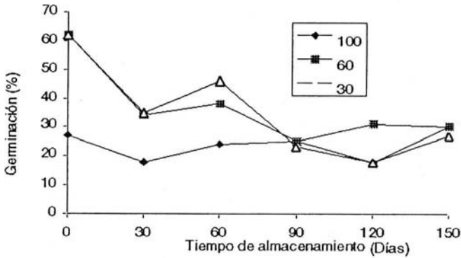
Figura 1. Germinación de Croton lechleri por efecto de la intensidad de luz y tiempo de almacenamiento.
