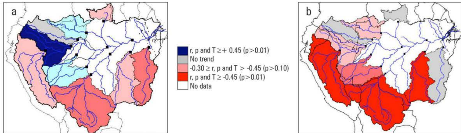
Figura 1. Coeficientes de correlación de Pearson ( r ), Spearman ( p ) y Kendall ( T ) entre la escorrentía y el tiempo (1974-2004) en las subcuencas amazónicas para (a) los valores máximos anuales y (b) los valores mínimos. Los valores por encima de 0.30 son significativos al nivel de 90%, aquellos por encima de 0.45 son significativos al nivel de 99%. Los colores indican la señal y la fuerza de la tendencia: rojo (tendencia negativa) y azul (tendencia positiva). Adaptado de Espinoza et al., [2009b].
