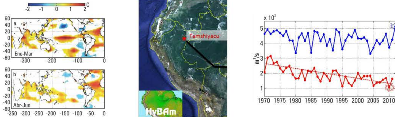
Figura 3. Anomalías de la temperatura superficial del mar (SST) durante a) Enero – Marzo y b) Abril-Junio de 2010 (expresado en °C). Solamente los valores más grandes que 2x la Desviación Standard son graficados. Adaptado de Espinoza et al. [2011]. c) Evolución de los caudales en el río Amazonas en la estación hidrométrica de Tamshiyacu (40km aguas arriba de Iquitos) durante el periodo 1970-2012. Línea azul: caudales durante el periodo de aguas altas (marzo-mayo). Línea roja, caudales durante el periodo de estiaje (agosto-octubre). Se muestran los valor extremos históricos: el más bajo ocurrido en septiembre 2010 y el más alto en abril 2012. Fuente: Espinoza et al. [2013].
